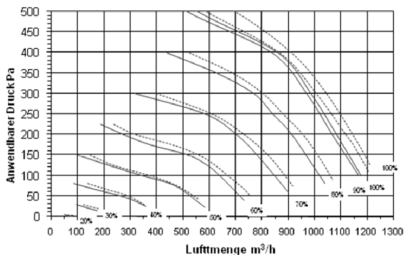
PEGASOS Eco ECE ZU- und ABLUFT Leistungskurven mit EU5 Taschenfilter
