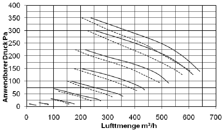
Pelican Eco ECE ZU- und ABLUFT Leistungskurven mit EU5 päsfilter
